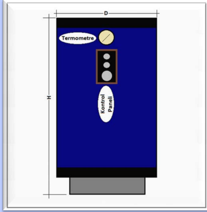
Çift Serpantinli Boyler / Boyut Şeması
