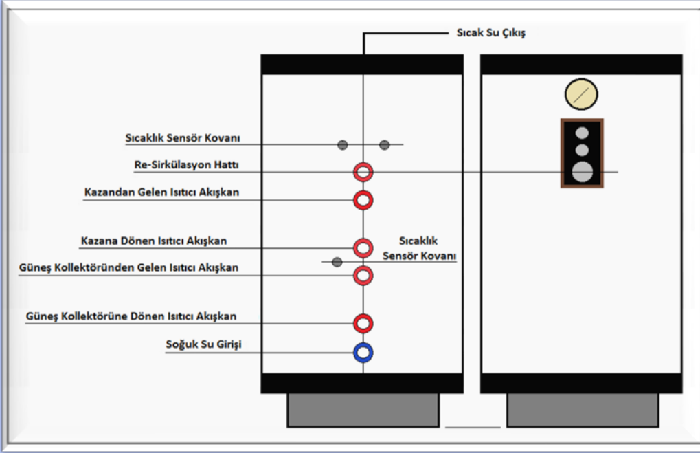
Çift Serpantinli Boyler / Tesisat Bağlantı Şeması
